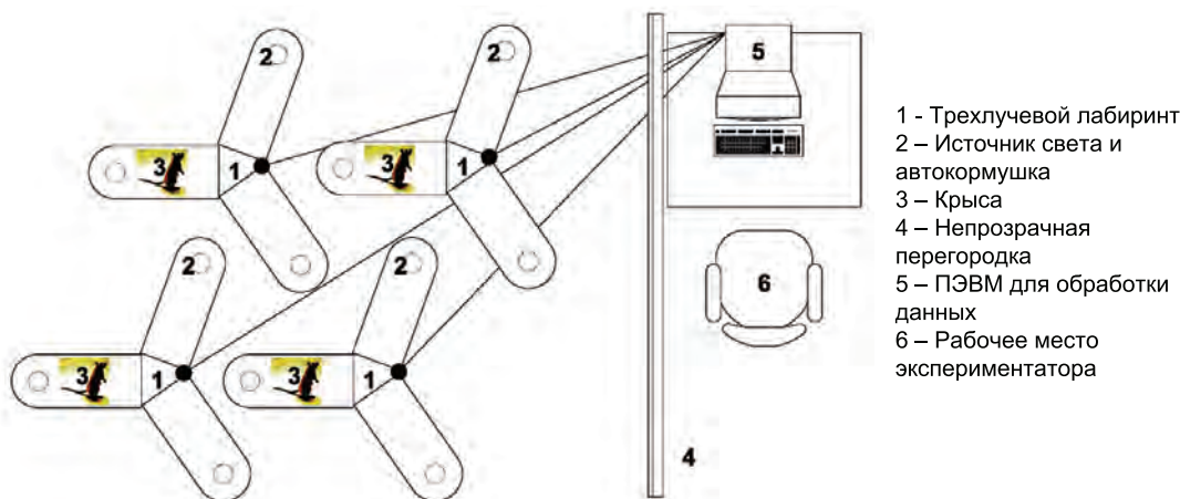
Рис. 1. Схема экспериментального комплекса «Трехлучевой лабиринт».
